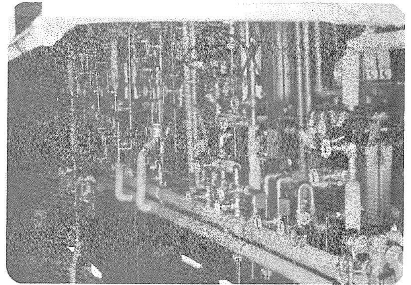
تصویر ۵۱. کارخانه صنایع اریشیم) مراحل مختلف خنده کردن و خشک کردن ببله
