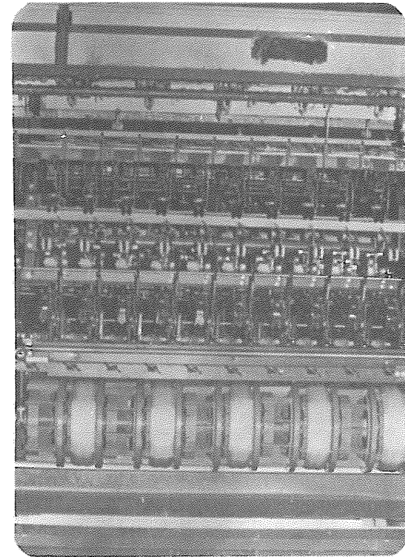
تصویر ۵۵. کارخانه صنایع ابریشم (مراحل مختلف کلاف کردن نخهای ابریشمی)
