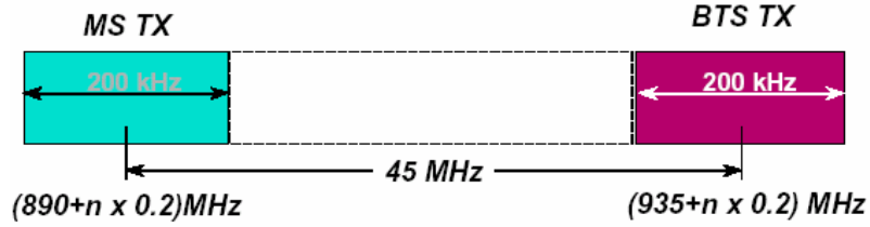
شکل (1-4): فاصله فرکانسی بین مسیر Downlink و Uplink
