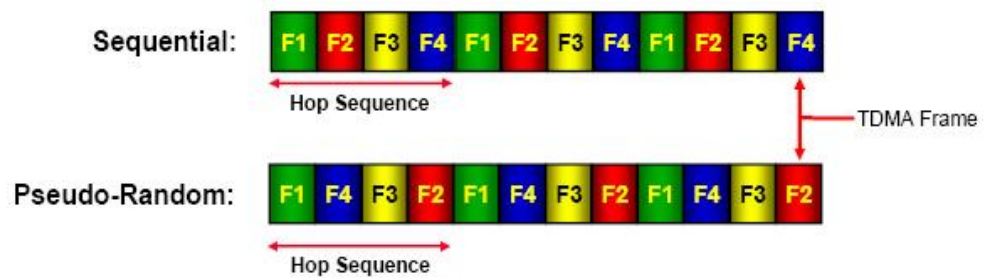
شکل (4-2): نوع پرش فرکانسی
