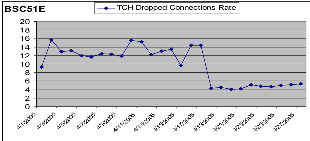
شکل (9-1): بهبود درصد قطعی مکالمات در کل BSC
