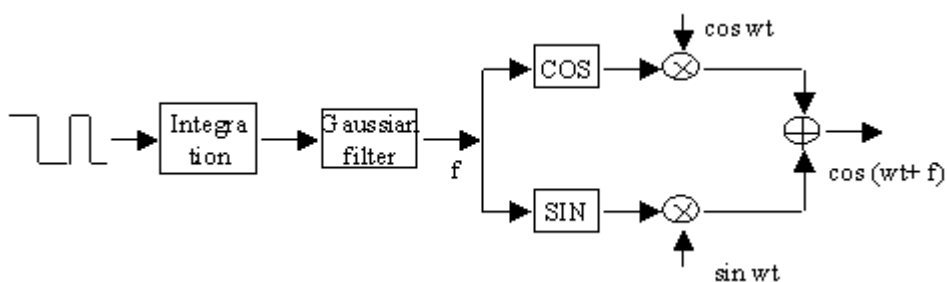
شکل (1-7): دیاگرام مدولاسیون GMSK
