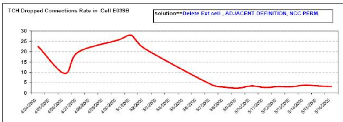
شکل (9-5) : نمودار بهبود درصد قطعی مکالمات با تصحیح لیست همسایگی
