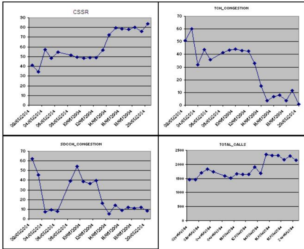
شکل (9-2): نمودار های بهبود KPI با فعال کردن فیچر Half Rate
