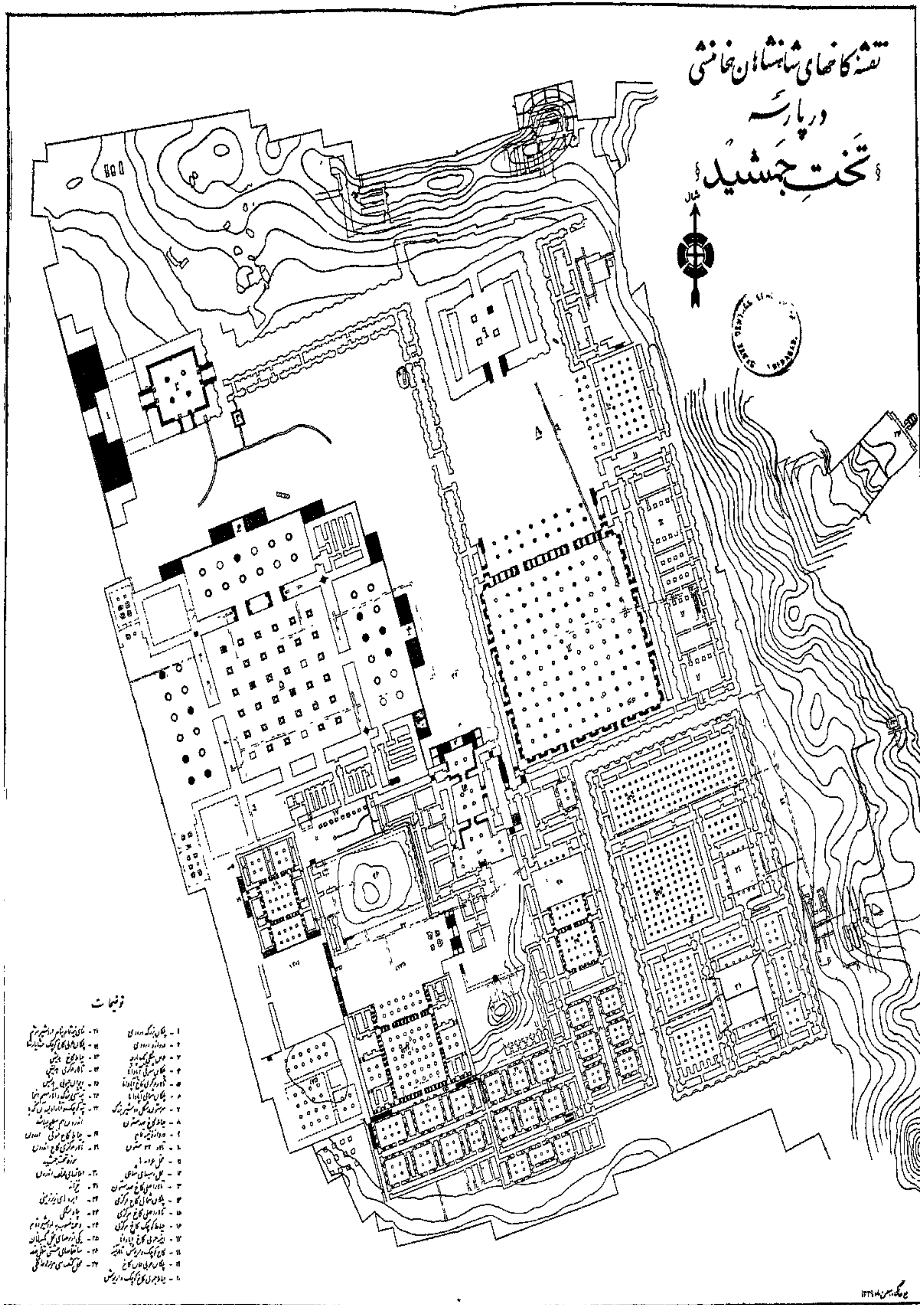
نقشه کامل آثار تخت جمشید که در بهمن ماه ۱۳۲۹ بوسیله آقای علی حاکی بازرسی فنی باستان شناسی ترسیم گردیده است مقیاس ۱/۱۷۵۰
