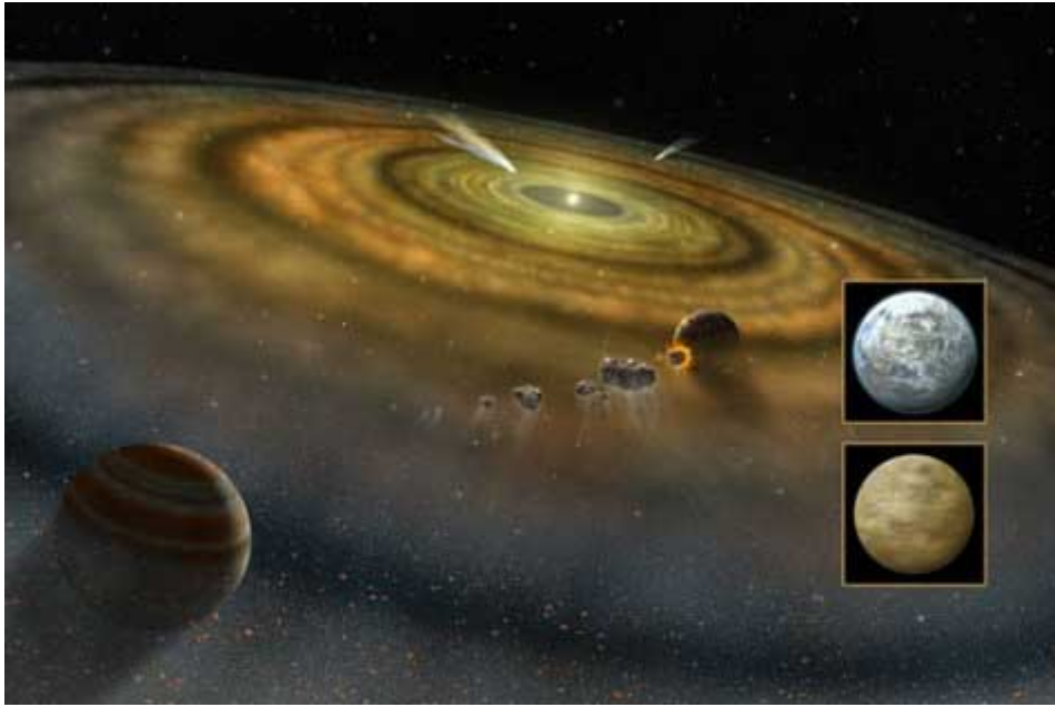
شکل (۵ - ۲) تصویری تخیلی از تشکیل یک سیستم ستاره ای نظیر سیستم خورشیدی ما در اطراف ستاره بتا پیکتوری Beta-Pictoris
